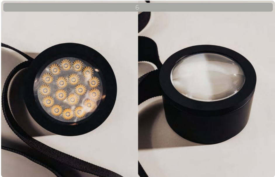
6 Close and magnetically seal the module by inserting the desired light solution from the available options. Chiudere e sigillare magneticamente il modulo inserendo la soluzione di luce desiderata tra le opzioni disponibili.
